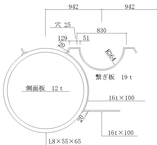
受台詳細図
