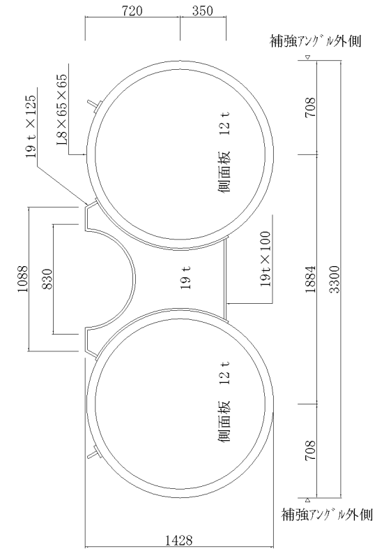
正面図
