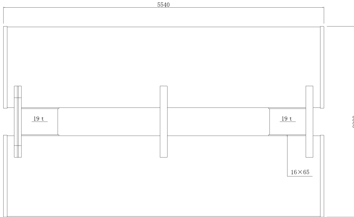
平面図
